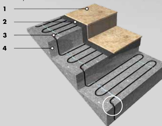
detail přechodu hrany schodu
